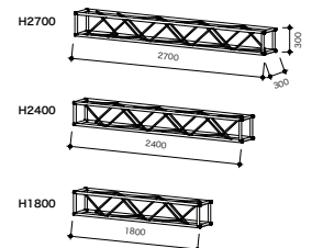
トラス
